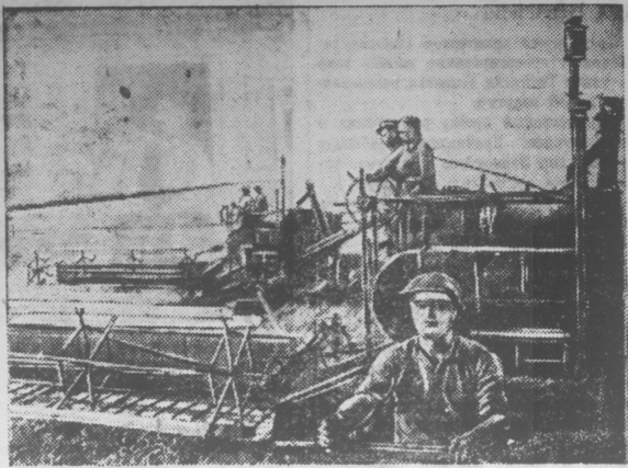
Комбайнер Ново-Расшеватской МТС Ново-Александровского района т. Аубенцов сцепом двух «Сталинцев» убрал 1610 гектаров колосовых. Фото О. ПОЖАРСКОГО
