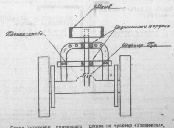
Схема установки привода шкива на трактор «Универсал».
